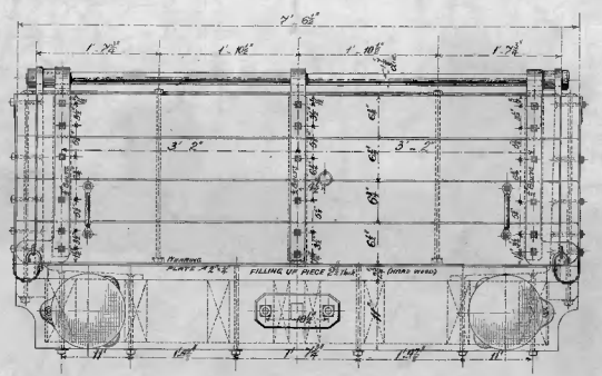
— END ELEVATION —
